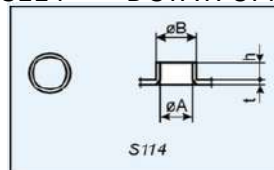
STAZ. B – ESTRUS. FILETT. S114 - B STAT. UPFORM BURRING S114
